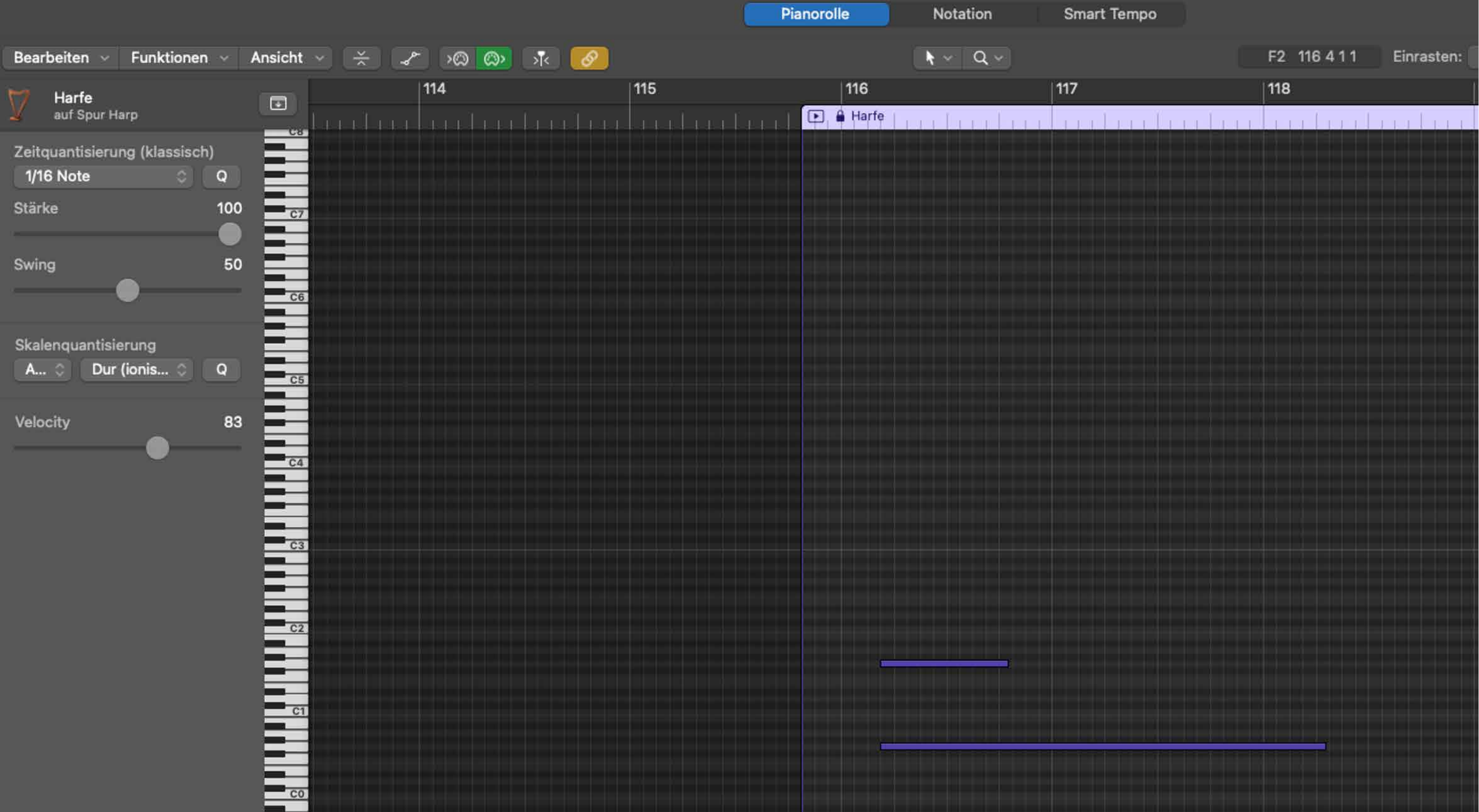
Abb. 1: Beispiel eines Harfenglissandos im MIDI-Bereich von Logic Pro. Dargestellt mit nur zwei einzelnen MIDI-Events wird hier das Softwareinstrument so getriggert, dass ein gesamtes Aufwärtsglissando ausgeführt wird (Screenshot der Autorin, 15.6.2025).
